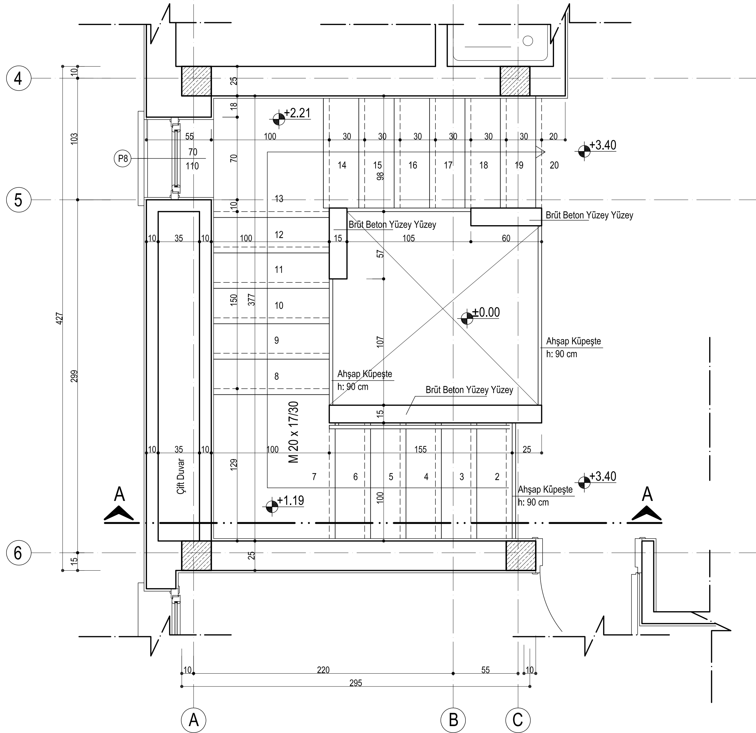
I. KAT PLANI ÖLÇEK:1/20
