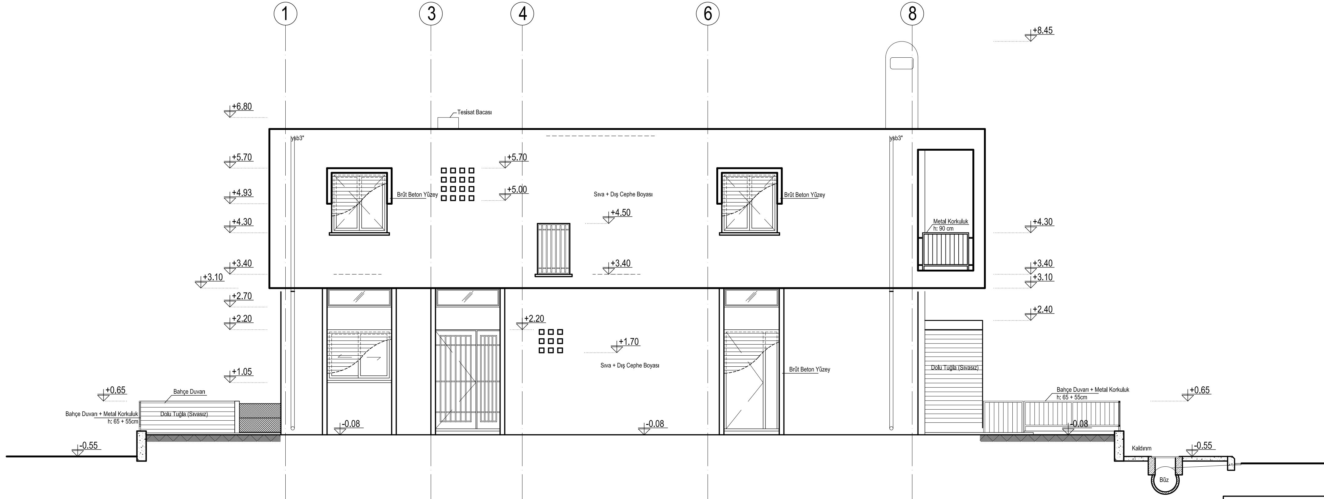
GÜNEY CEPHESİ ÖLÇEK:1/50
