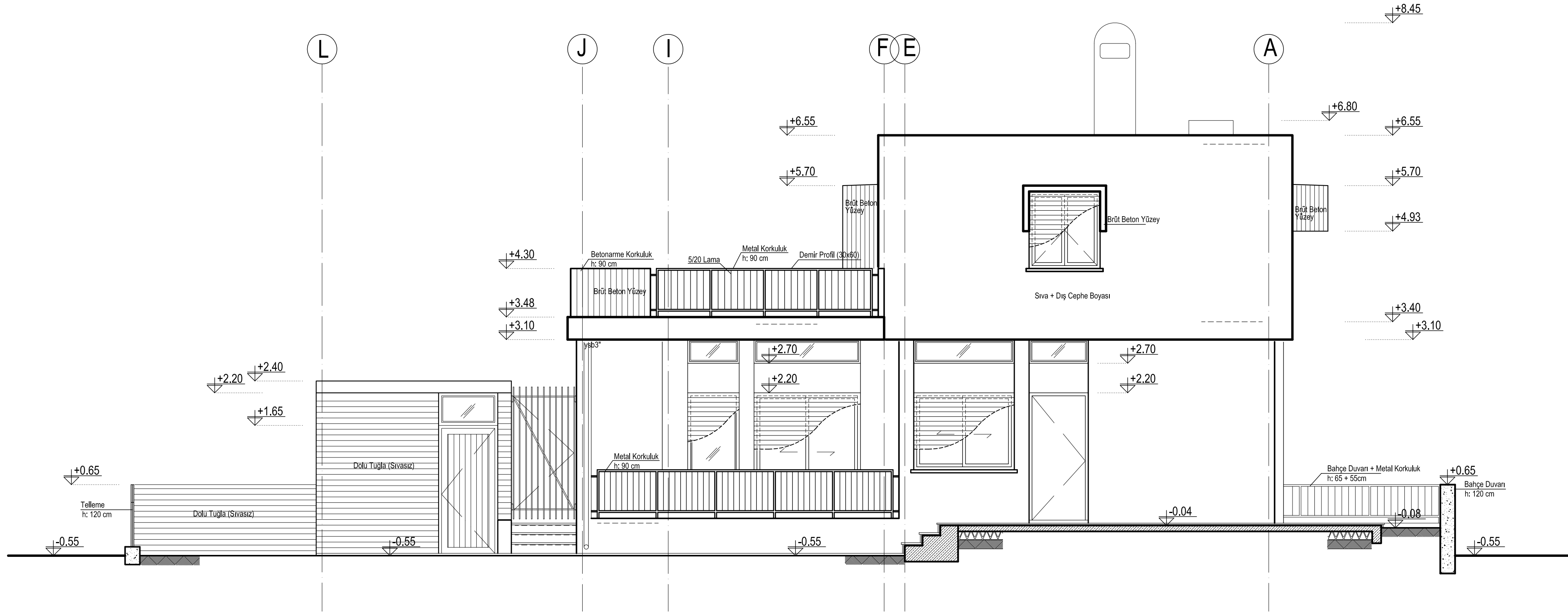
GÜNEY CEPHESİ ÖLÇEK:1/50
