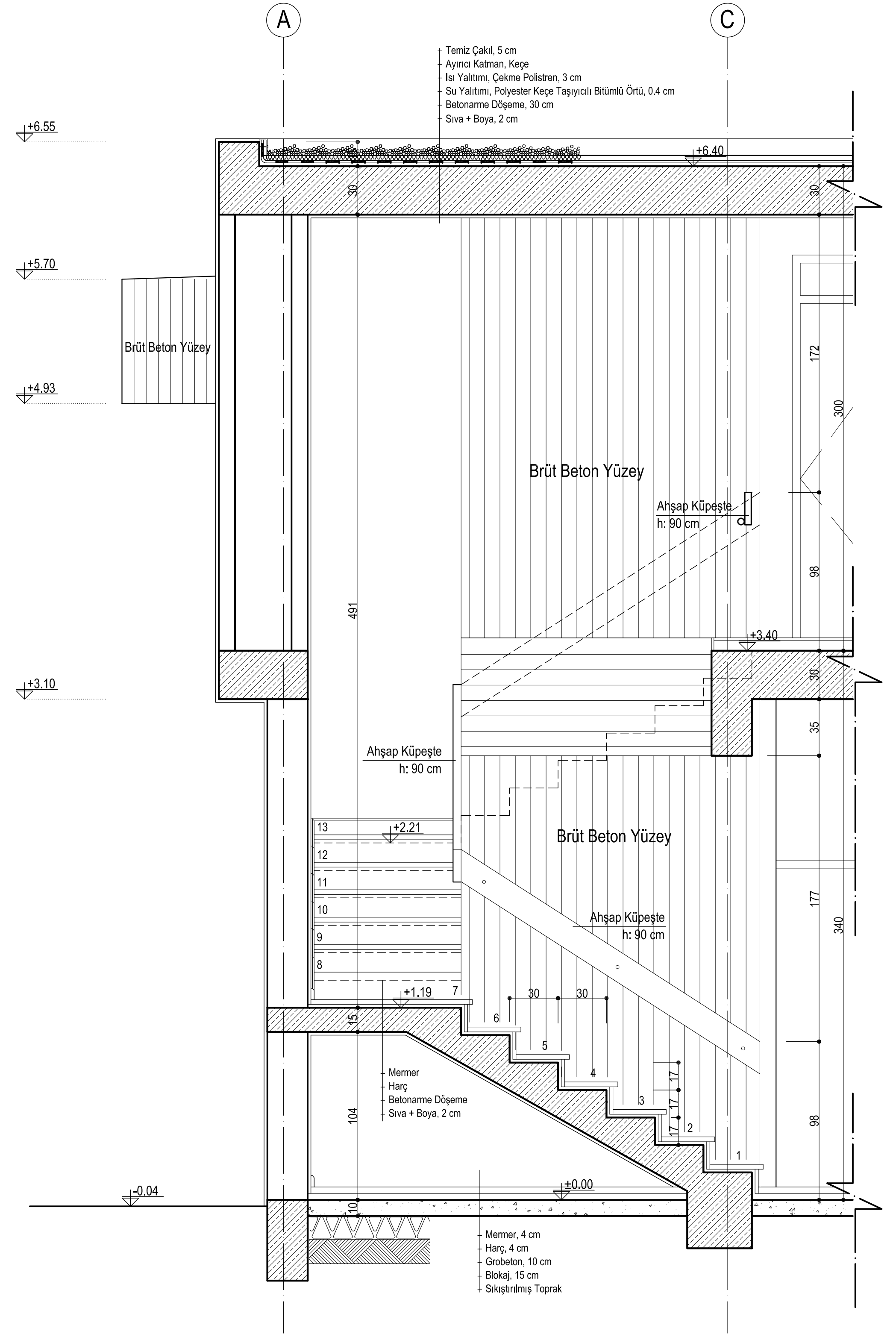
A-A KESİTİ ÖLÇEK:1/20
